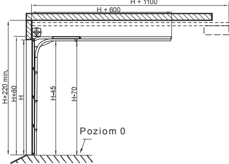
System: Sprężyny skrętne z przodu (minimalne nadproże 220 mm)
