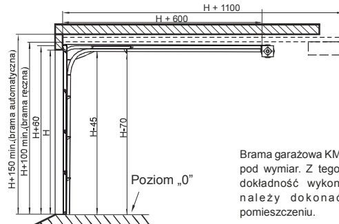
System: Sprężyny skrętne z tyłu (niskie nadproże) (brama ręczna minimum 100 mm nadproża, brama automatyczna minimum 150 mm nadproża)
