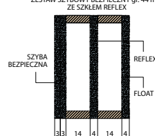
DOSTAWKA ZESTAW SZYBOWY BEZPIECZNY gr. 44 mm ZE SZKŁEM REFLEX
