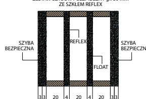
ZESTAW SZYBOWY BEZPIECZNY gr. 80 mm ZE SZKŁEM REFLEX
