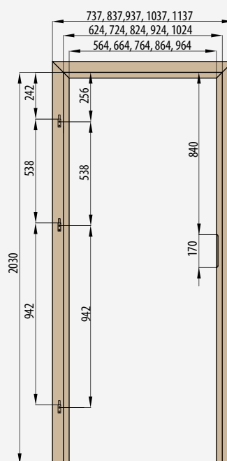
OŚCIEŻNICA NAKŁADKOWA
