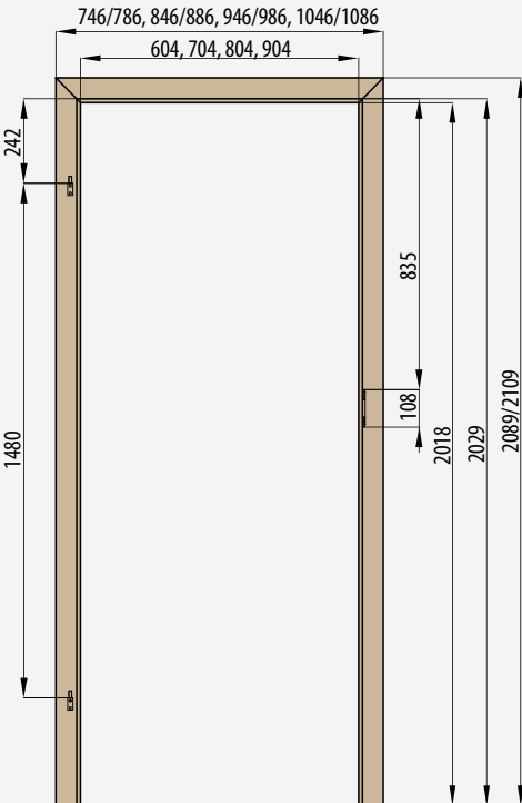
OŚCIEŻNICA REGULOWANA DO DRZWI SZKŁANYCH opaska 6 cm/opaska 8 cm
