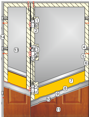
KMT PLUS 54 - dostawka nie otwierana
