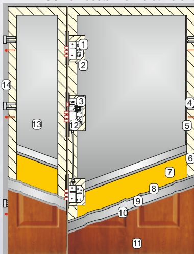
KMT PLUS 75 - dostawka nie otwierana
