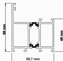
Profil progów ENERGY 60
