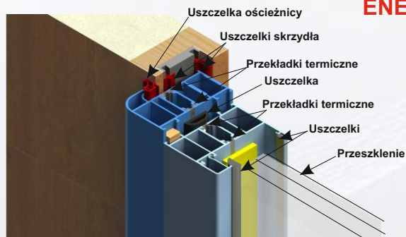
SKRZYDŁO KMT PLUS 75 passive PROFIL OŚCIEŻNICY ENERGY 90 + PROFIL NAŚWIELTA
