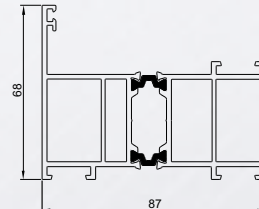
Profil progów ENERGY 90
